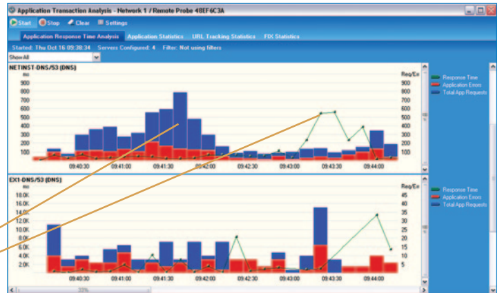
Analyses des transactions applicatives
